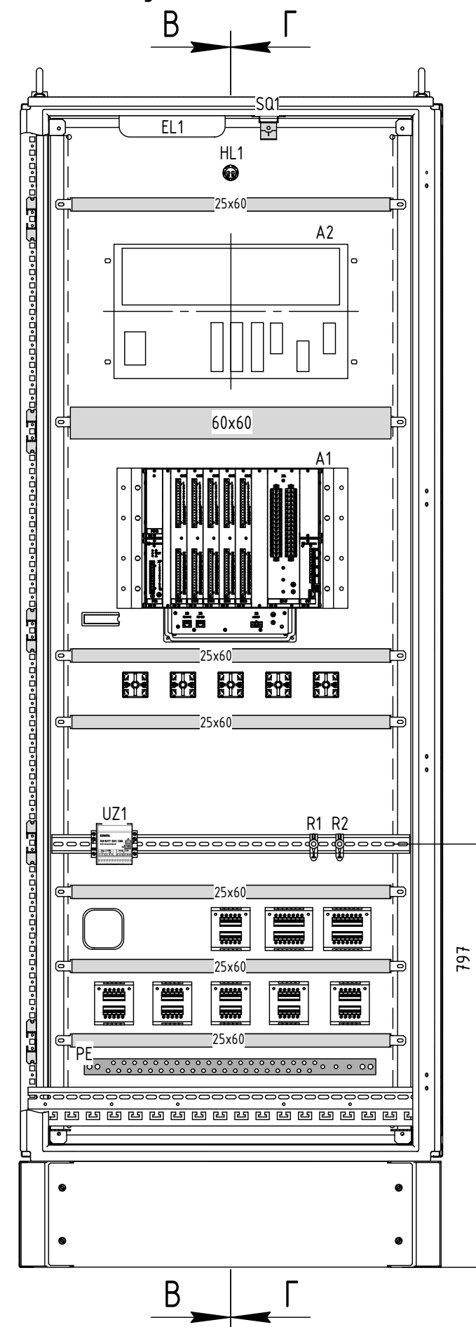
Вид сзади Дверь, ряды зажимов и вертикальные короба условно не показаны
